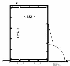
Plattegrond
