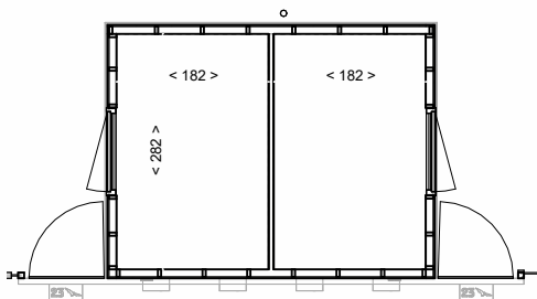
Plattegrond
